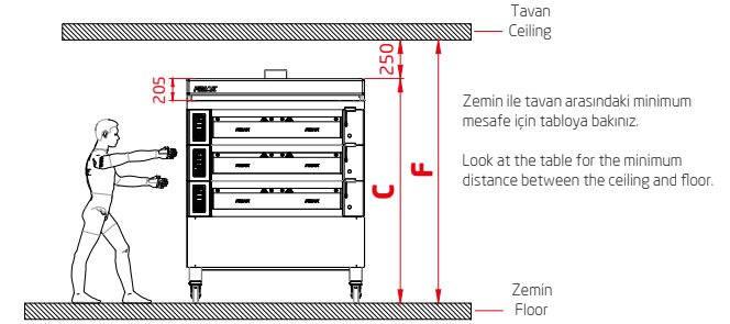
Ön Görünüş Front View
