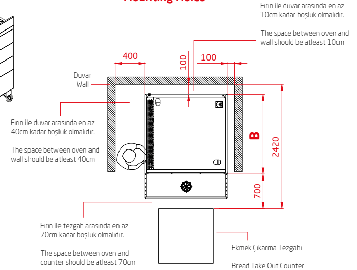
Montaj Boşlukları Mounting Holes
