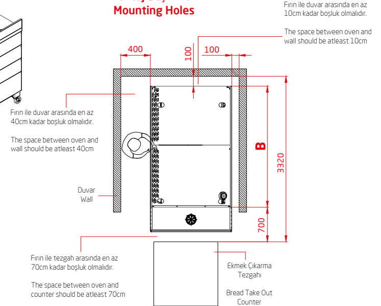
Üst Görünüş Top View
