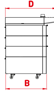
Sol Yan Görünüş Left Side View
