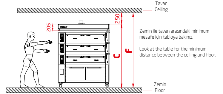
Ön Görünüş Front View
