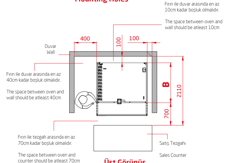
Montaj Boşlukları Mounting Holes
