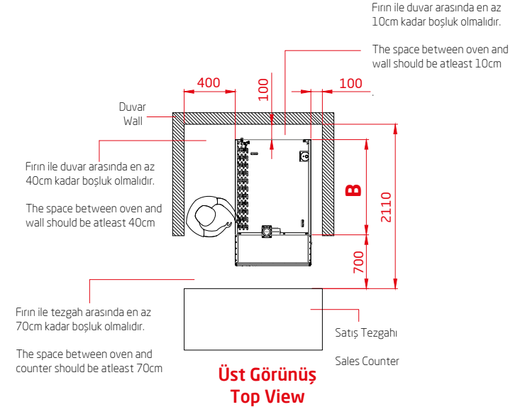
Montaj Boşlukları Mounting Holes
