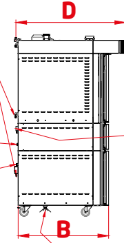
Sol Yan Görünüş Left Side View
