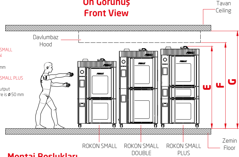
Montaj Boşlukları Mounting Holes
